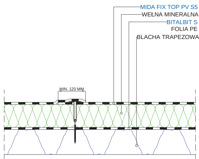
Rys. 14 System jednowarstwowy na podłożu z blachy trapezowej
