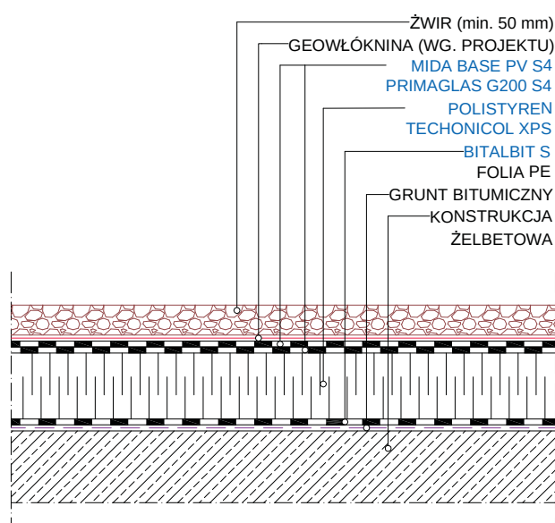
Rys. 20 System balastowy
