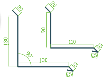
Zapora przeciwniegiwa
