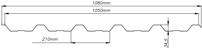
T35/1050 - PROFIL DACHOWY
