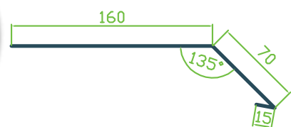
Pas nadrynnowy
