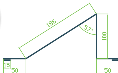
Pas nadrynnowy
