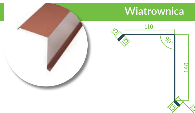
Wiatrownica GRANDE
